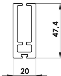
Dolní profil FZ 47 (3-03058-PU11)
